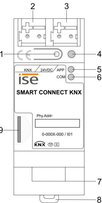
Abbildung 1: Geräteaufbau Figure 1: Device design Afbelding 1: Opbouw van het apparaat Figura 1: Struttura dell'apparecchio Figura 1: Estructura del dispositivo Figure 1: Structure de l'appareil
